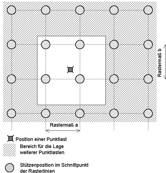
Abbildung 1: Mindestabstand möglicher Lastenleitungsunkte bei Systemböden
