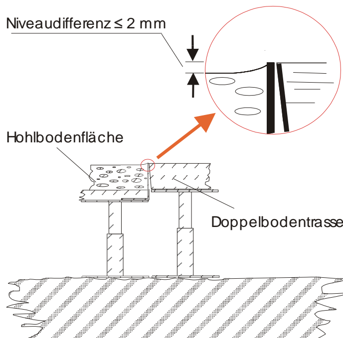
Skizze: Niveaudifferenz bei Doppelbodentrassen
